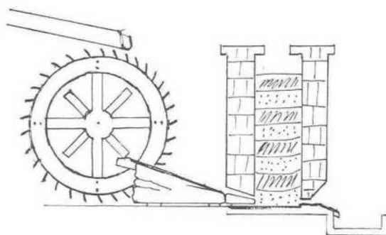
Indrez d'ina cularia
