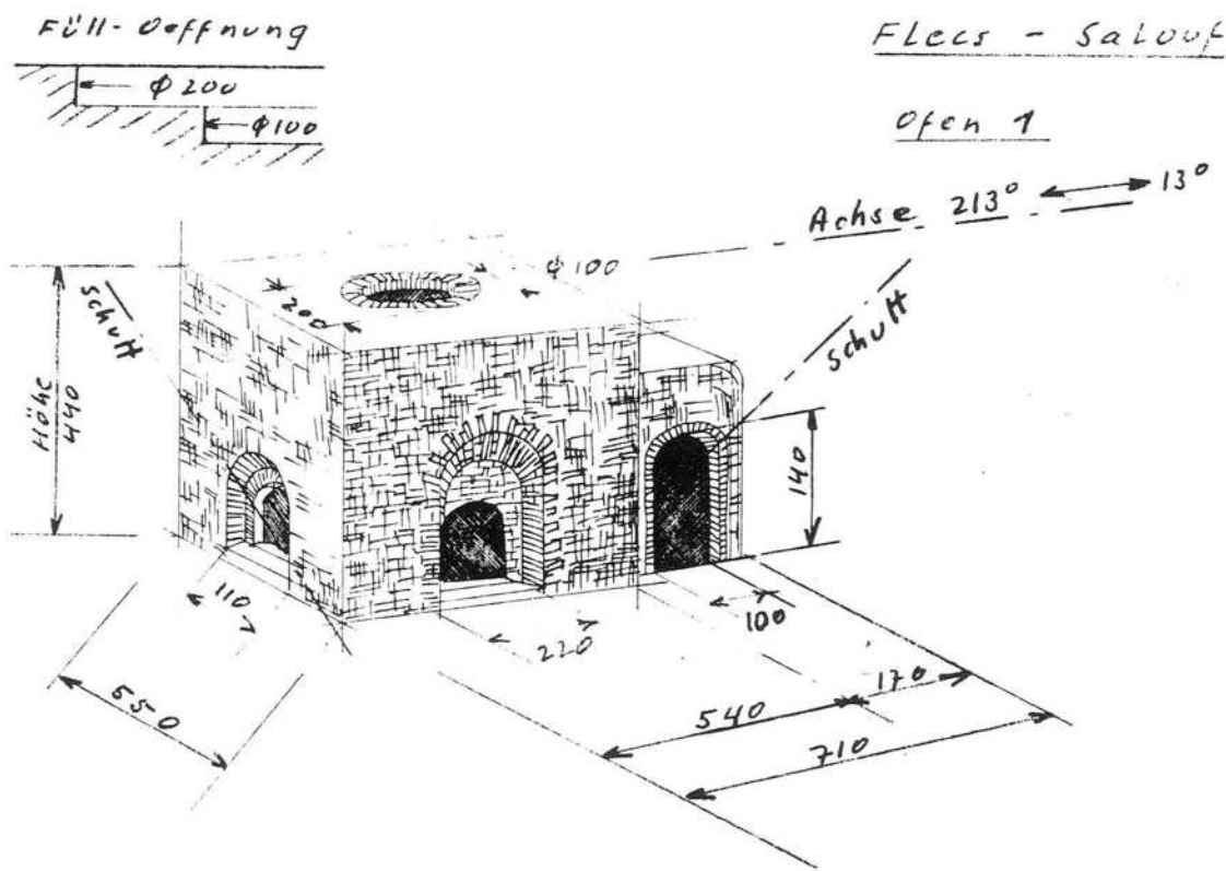
SKIZZE von Ofen 1 nach V. Dietrich (1972)
