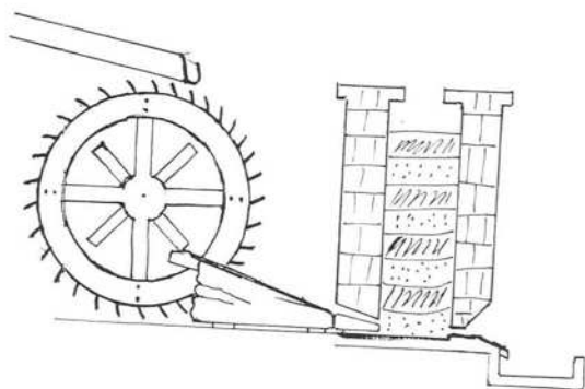
Fuorn per alquantar il plom
