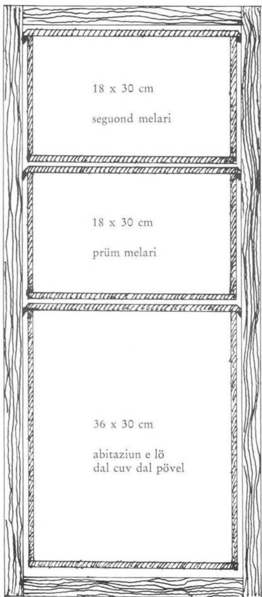
Tagl transversal da la chaista tip svizzer
