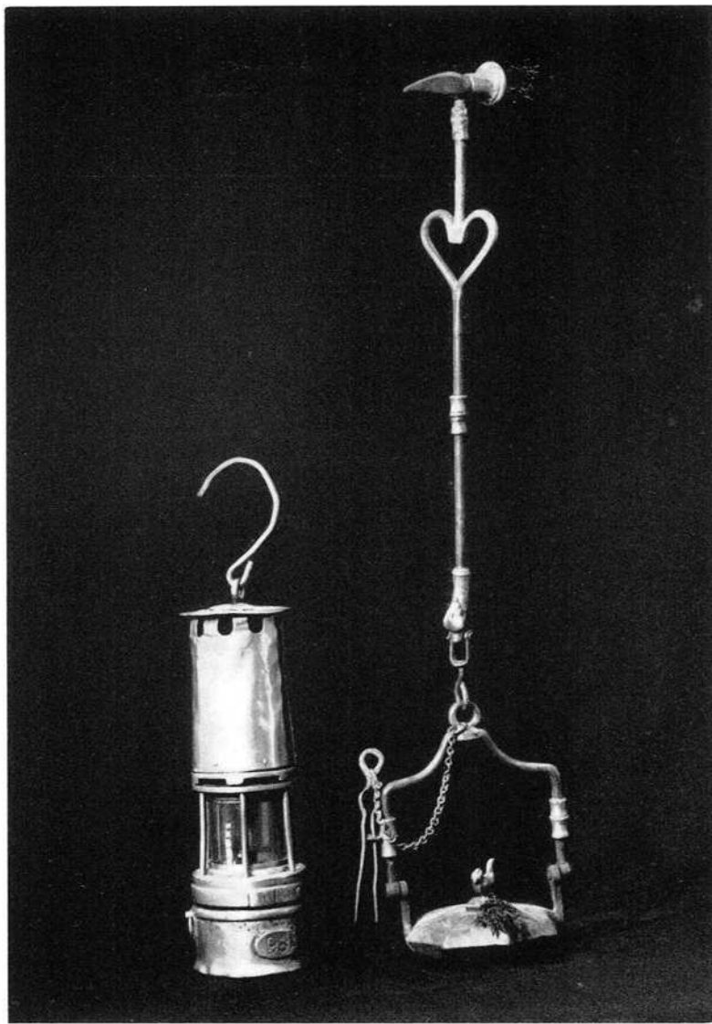
Seniester : lampa de segirezia per miniers, sistem Davy, per benzin, 19. tschentaner. Dretg : lampa de minier, per ieli. Duvrada el vegl tunnel dil Hauenstein, 1853.
