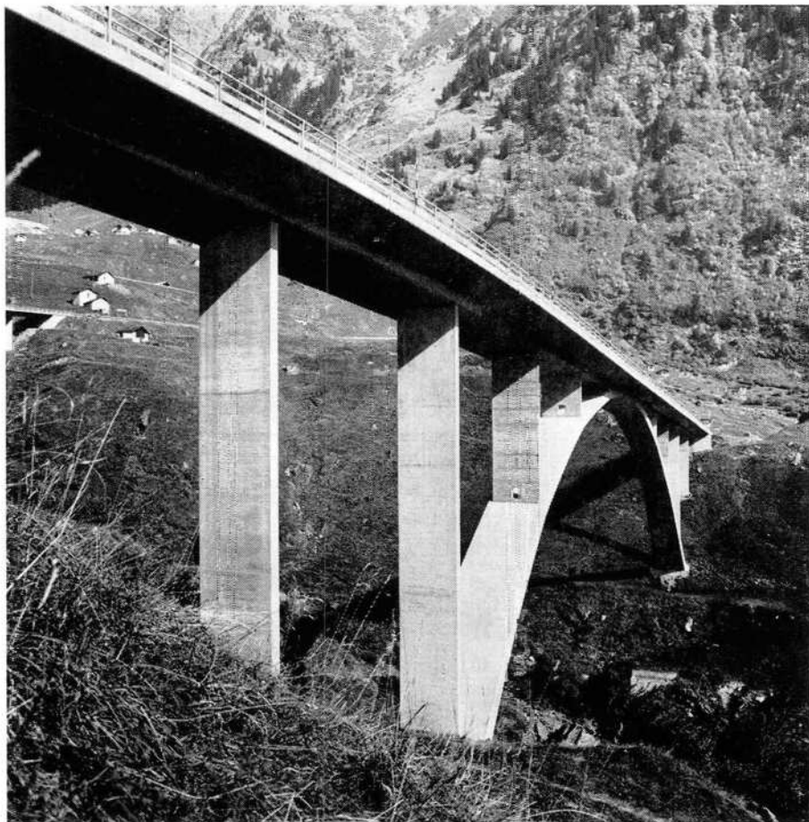
Ponte Nanin en sia construcziun de beton razionala. Ils pilasters, mo cunzun ils dus peis digl artg ston esser bein sfunsai e fundai. Ei tucca de puder tier grep. (Foto Uff. de constr. bassa: L. Cramer)
