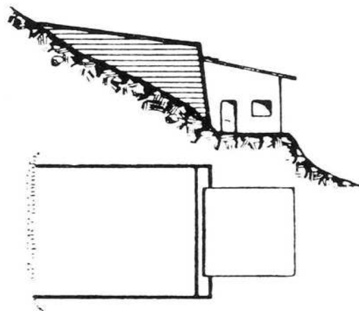
Foto 14 Rempar «Ebenhöch» — La part encunter mun dil baghetg che duei vegnir schurmegiaus empleinan ins tochen tier il tetg cun tratsch e crappa. La lavina vegn menada sur il baghetg ora.
