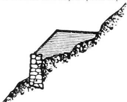
Fig. 1b Terrassa cun pei de mir — Il mir schetg al pei della terrassa aulza siadora quella empau pli fetg. Quei tip de terrassa mischedada han ins entschiet a baghegiar entuorn 1900 ad Elm/Glaruna.
