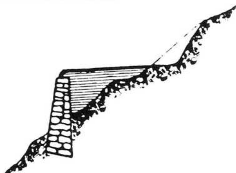
Fig. 1c Terrassa cun in mir — In ferm e gries mir schetg ord sauna crappa cun bien fundament fa la terrassa pli lada e pli aulta. Cheutras vegn la neiv retenida meglhier.
