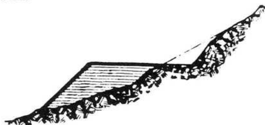
Fig. 1a Terrassa — La via de 50—100 cm ladezia ei stada ina dellas empremas lavineras. La scarpa davontier ei rinforzada cun tschespets e plattas-crap.
