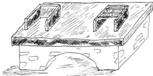
Platta a la veglia cun furnels per accoglier il fö e tgnair ils tests. Il furnel a dretta ais muni d'una graddella fatta our da bachettas da fier. (Disegnà tenor descripziuns fattas a Lavin e Guarda).
