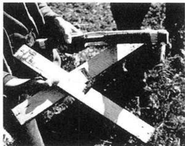
Las parts della roda: alas adencrusch, arver scalpraus tras, il bintgun e las cavrinas. (Foto A. Maissen)
