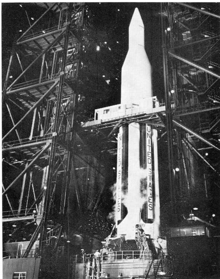
Ina racheta dil tip Saturn ord la seria d'emprova durant la cargada dil carburont. Seniester la tuor de montascha, in monster carrabel, dretg la propria rampa de sittar. Igl um seniester della racheta, sper il tschabergal, dat in'idea della grondezia dil projectil. — Foto spk — Berna.
